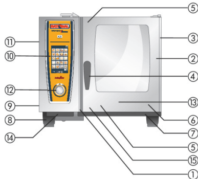
Tischgerät BakkingLine
